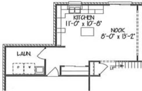
OPTIONAL LAUN. RM LAYOUT ADDS 72 SF
